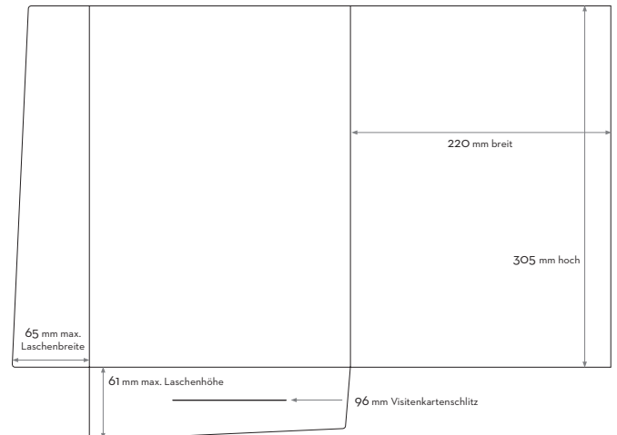
Mappe 6 ohne Füllhöhe - offenes Format 505 x 367 mm Werkzeugnummer: W 105/07
