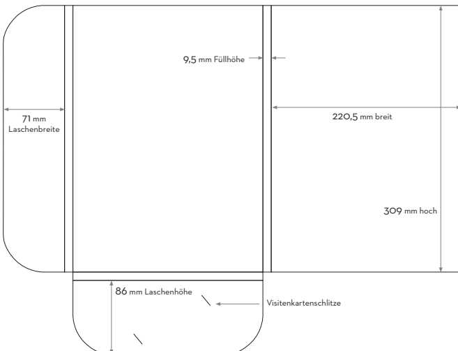
Mappe 5 mit Füllhöhe - offenes Format 532 x 404,5 mm Werkzeugnummer: W 76/13
