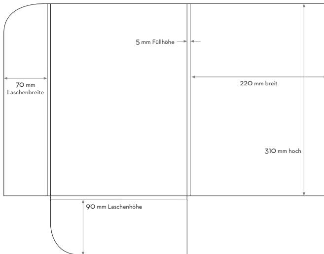
Mappe 3 mit Füllhöhe - offenes Format 520 x 405mm Werkzeugnummer: W78/03
