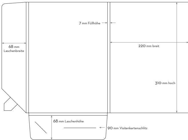
Mappe 1 mit Füllhöhe - offenes Format 522 x 385mm Werkzeugnummer: W 6/93
