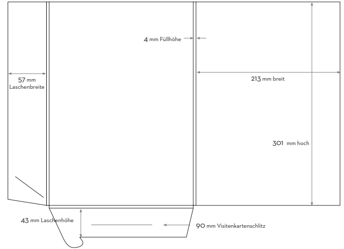
Mappe 2 mit Füllhöhe - offenes Format 491 x 363mm Werkzeugnummer: W251/98
