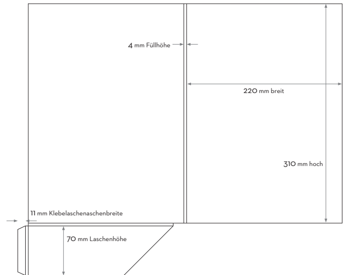
Mappe 4 mit Füllhöhe - offenes Format 459 x 384 mm Werkzeugnummer: W107/11
