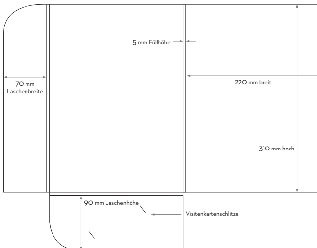
Mappe mit Füllhöhe - offenes Format 520 x 405mm Werkzeugnummer: W78/O3
