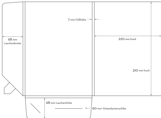
Mappe mit Füllhöhe - offenes Format 522 x 385mm Werkzeugnummer: W 6/93
