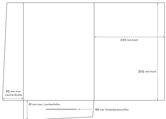
Mappe ohne Füllhöhe - offenes Format 505 x 366 mm Werkzeugnummer: W 105/07
