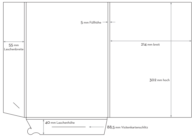
Mappe mit Füllhöhe - offenes Format 493 x 347mm Werkzeugnummer: W37/13
