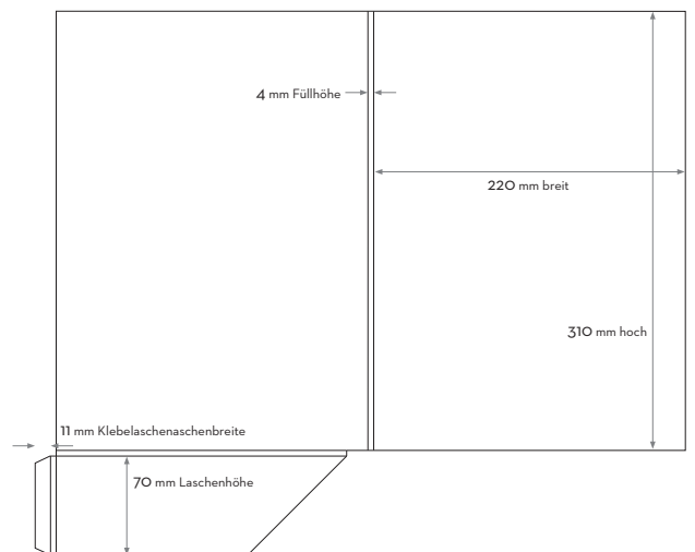
Mappe mit Füllhöhe - offenes Format 459 x 384 mm Werkzeugnummer: W107/11
