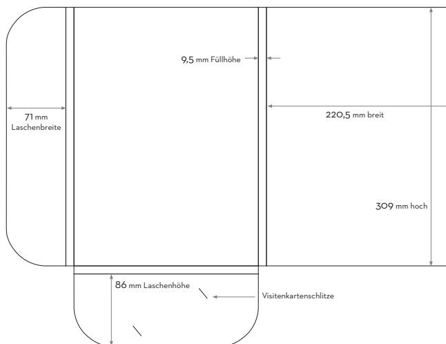
Mappe mit Füllhöhe - offenes Format 531 x 405,5 mm Werkzeugnummer: W 76/13
